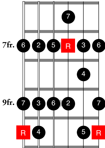
D Ionian
