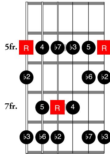
A Phrygian
